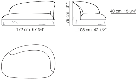
Divano / Versione con gonnella Sofa / Version with skirt
