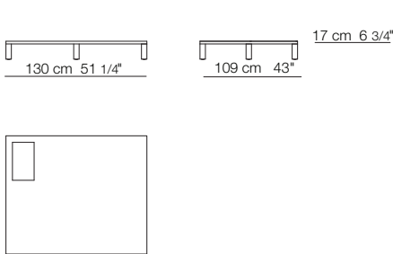
Tavolino Small table
