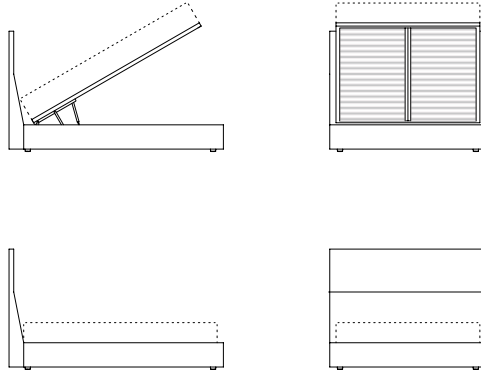
Everest Storage Bed Queen EVR100Q L 229cm W 167cm H 129cm / L 90" W 65¾" H 50¾"
