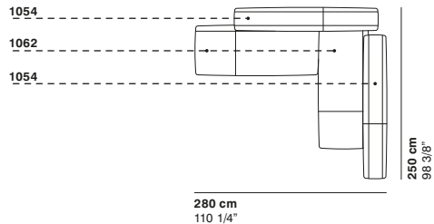
cod. SUI16DX / composition
