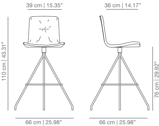
KLTBARTS swivel bar stool
