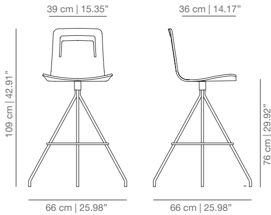
KLTBAR_R swivel bar stool
