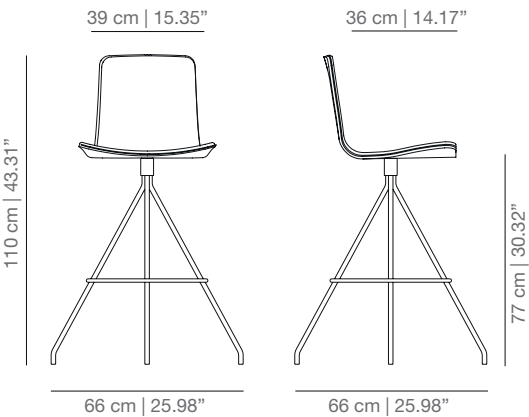
KLTBART swivel bar stool
