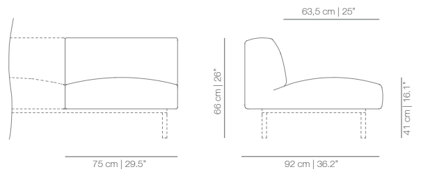
SISBP - LOW BACK MODULE
