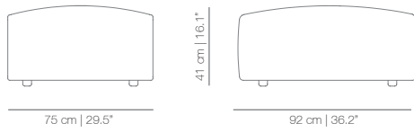
SISSR - BACKLESS MODULE
