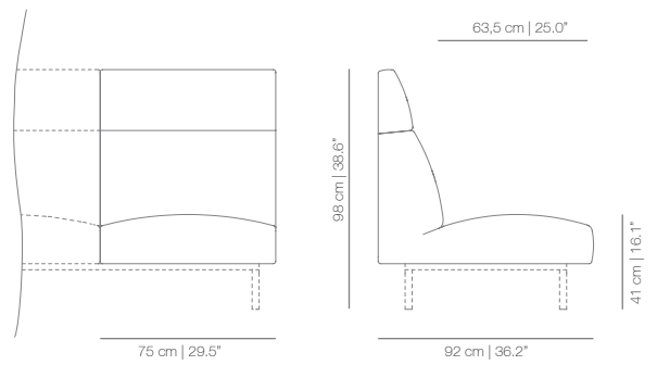
SISAP - HIGH BACK MODULE
